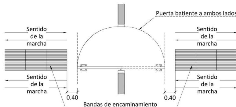
Banda de encaminamiento con puerta abatible a ambos lados
