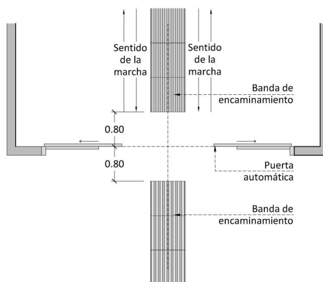
Banda de encaminamiento con puerta automática
