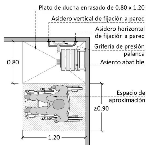
Asiento abatible
