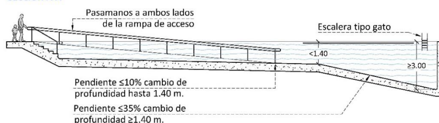
SECCIÓN A-A'
