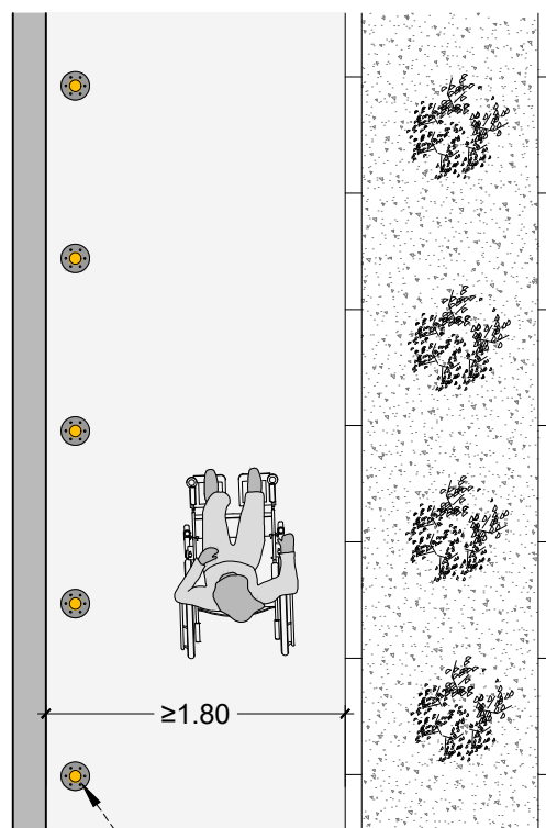
Luminaria empotrada a suelo con resalte \leq 4 mm.
