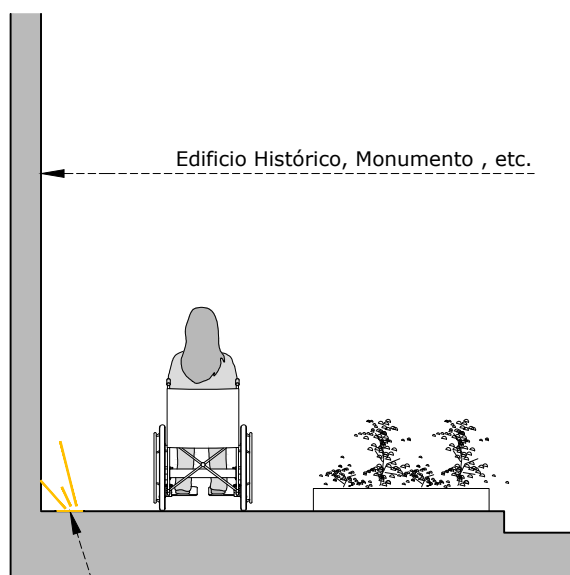
Luminaria empotrada a suelo con resalte \leq 4 mm, enfocada hacia el lateral para evitar deslumbramientos
